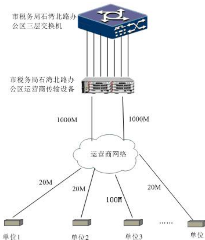
(2) 阳江市税务局石湾北路办公区至外部单位组网拓扑图
